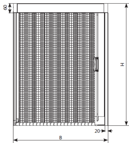
Montage: Fensternische
