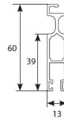
Rahmenprofil
