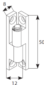
Scharnier – Aluminium (im Standard)
