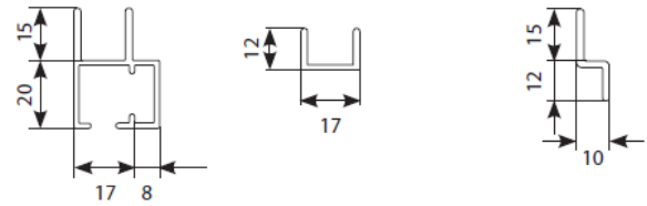
Laufschiene Typ C Laufschiene Typ B Laufschiene Typ A (Winkelprofil)
