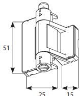
Scharnier - Selbstschließend (Aufpreis)
