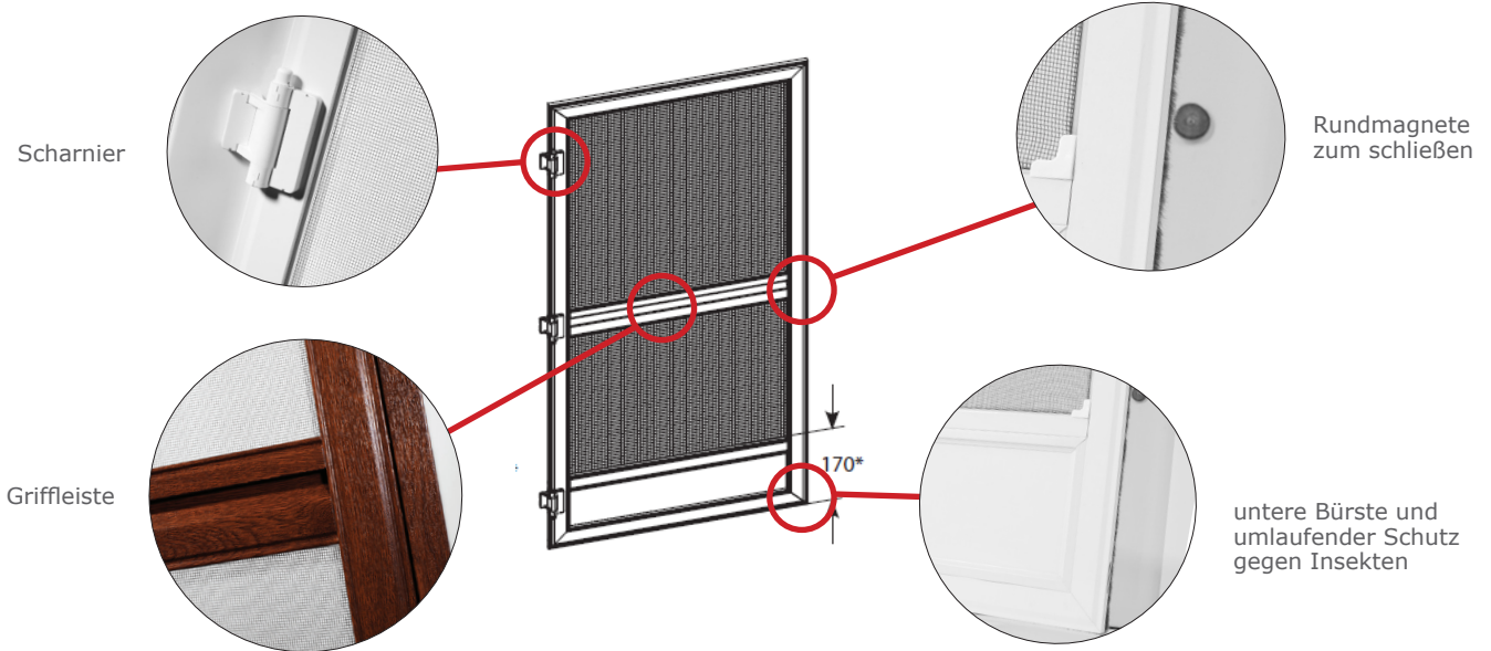
Scharnier - Aluminium (Im Standard)
