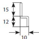
Laufschiene Typ A (Winkelprofil)
