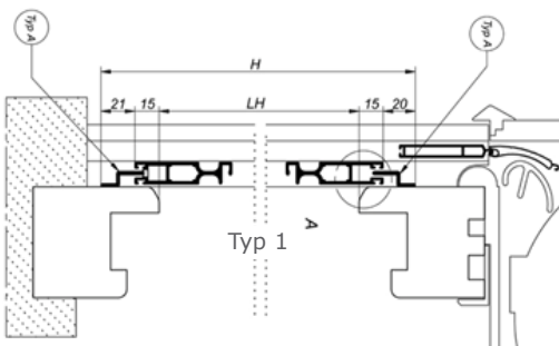
Laufschiene Typ A (Winkelprofil)
