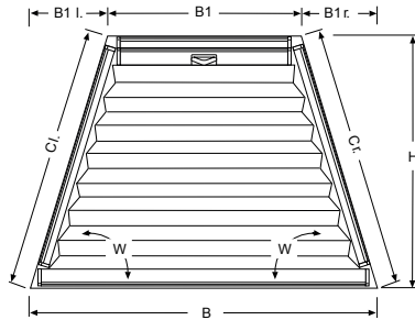
VS 7 Trapez Symmetrisch und asymmetrisch
