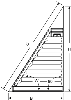
VS 10 Dreieck (1 Schräge)
