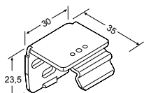
Wandträger 48200 grau 48201 weiß 48202 schwarz
