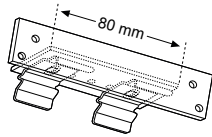
Befestigungsträger (VS 9) 80 mm 48245 grau 48246 weiß 48247 schwarz
