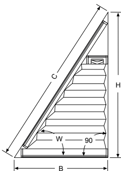
VS 10 D Dreieck (1 Schräge)
