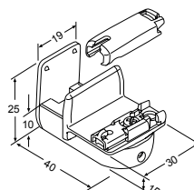
Klemmträger mit Spannschuh 48333 grau 48334 weiß 48335 schwarz
