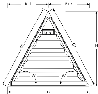
VS 9 D Dreieck Symmetrisch und asymmetrisch
