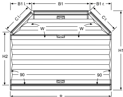
VS 6 SD Sechseck Symmetrisch und asymmetrisch, bei gleicher Höhe H2
