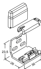
Winkel mit Spannschuh 48224 grau 48225 weiß 48226 schwarz
