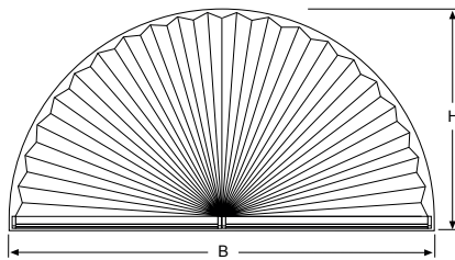
SR 1: Breite, Höhe (Radius = halbe Breite)
