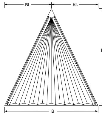
SD 3: Breite, Höhe, Schräge links, Schräge rechts
