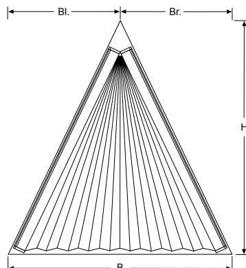
SDP 3: Breite, Höhe, Schräge links, Schräge rechts
