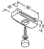
Verrastung Ø10 VS (empfohlen ab 100 cm Anlagenbreite) 48314 grau 48315 weiß 48316 schwarz
