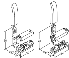
Glasleistenwinkel VS, Paar 48210 grau 48211 weiß 48212 schwarz VS 1, VS 3 u. VS SD 3 = max. Anlagenbreite 50 cm
