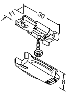
Spannschuh mit Verrastung 49141 grau 49142 weiß 49143 schwarz
