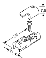
Spannschuh 48141 grau 48142 weiß 48143 schwarz
